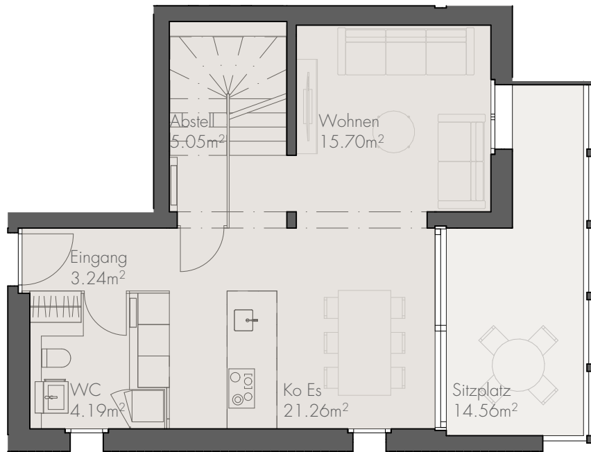
Obergeschoss
